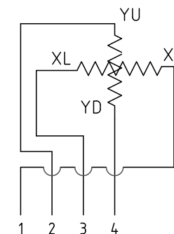
ピンアサイン
