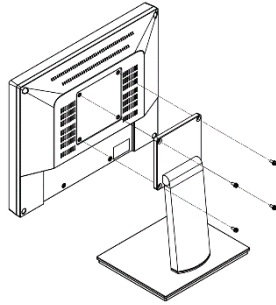
取付け図
